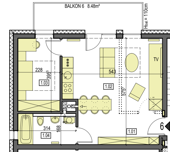
Rzut mieszkania 1:100
