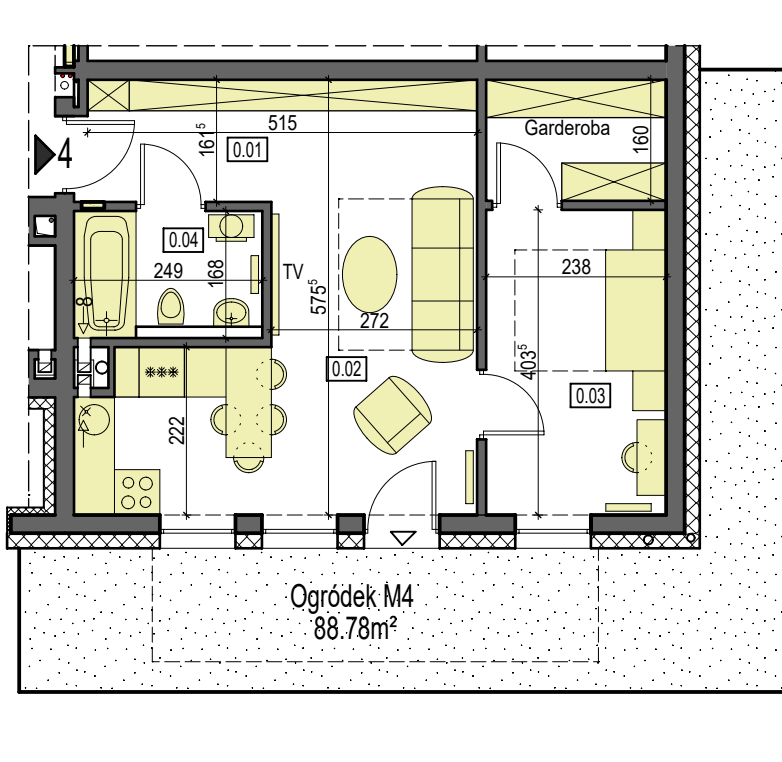
Rzut mieszkania 1:100
