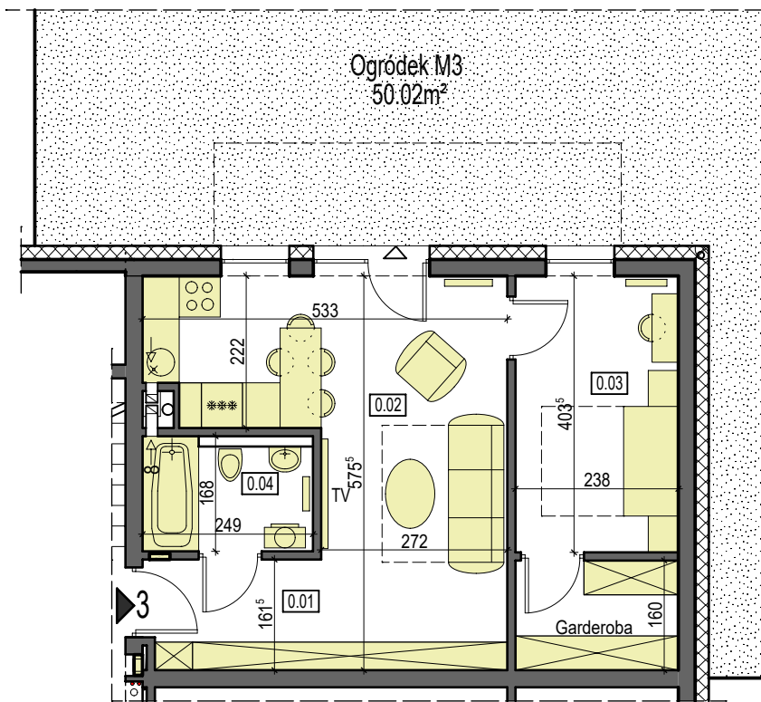
Rzut mieszkania 1:100
