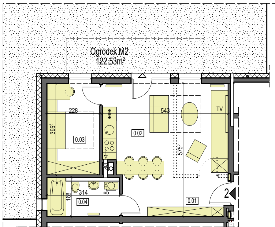
Rzut mieszkania 1:100
