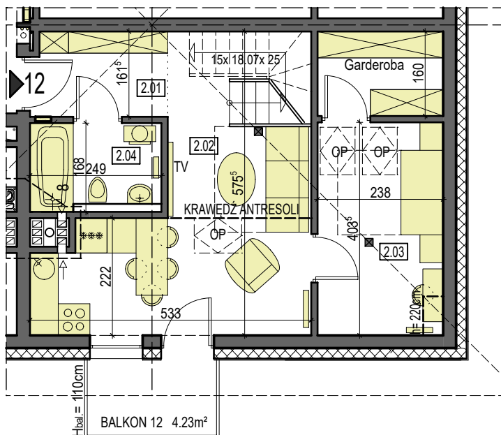
Rzut antresoli 1:200
