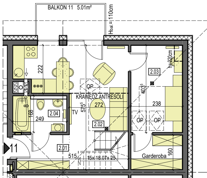
Rzut antresoli 1:200
