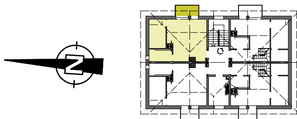
Rzut mieszkania 1:100
