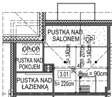
Rzut antresoli 1:200
